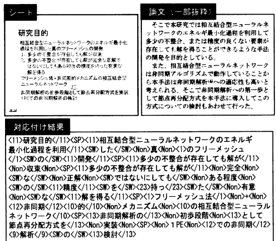
図 3 HMM による対応付け結果の具体例
