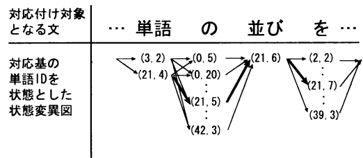
図 1 Jing の手法における状態変異図の具体例
