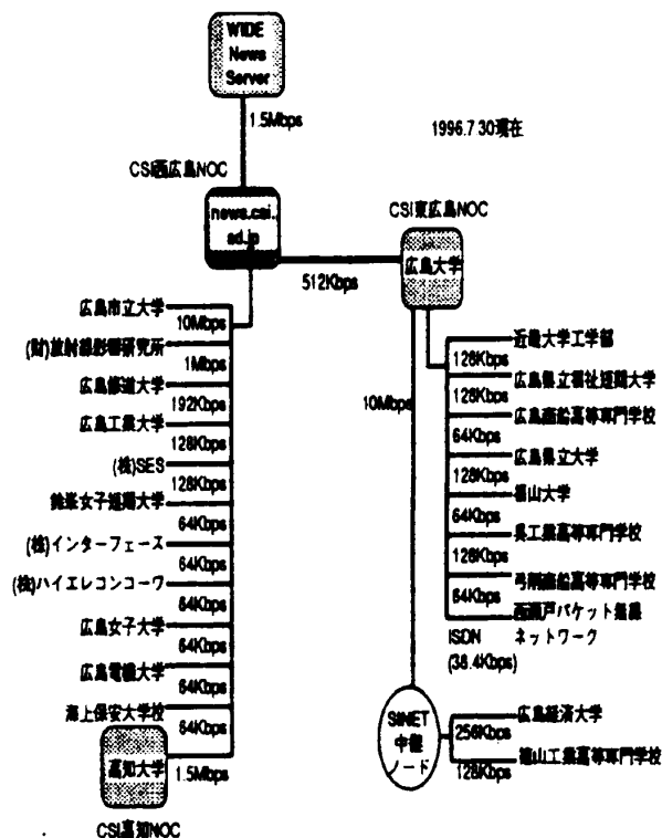
図 2: CSI のニュース接続関係
