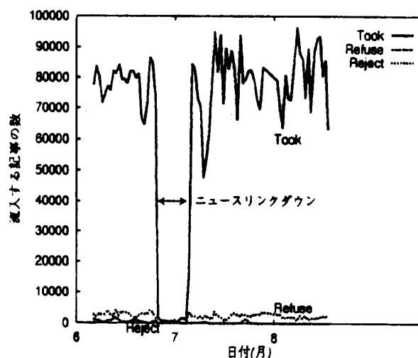
図 3: CSI1 次サーバの記事流量
