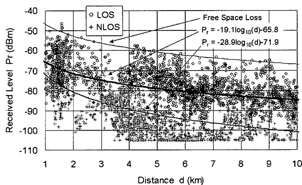
図 16 受信レベル距離特性 (送信局: Koi) Fig. 16 Received level characteristics (Koi).
