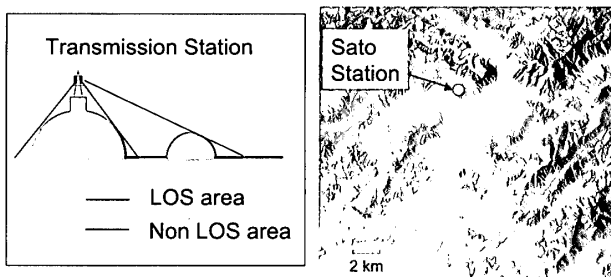
(a) Concept of terrain LOS (b) LOS simulation example 図 8 送信局からの見通しエリアの導出例
