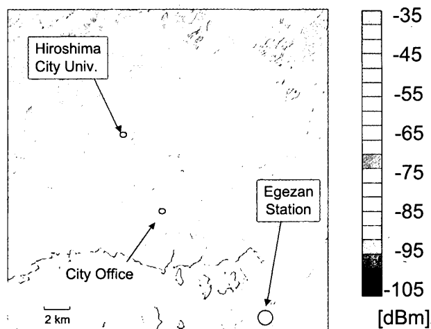
図 13 LOS 受信レベルマップ (送信局: Egezan)
