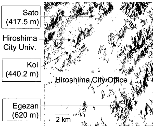
図 7 測定に用いた TV 放送波送信局の位置 Fig. 7 The position of transmission stations.
