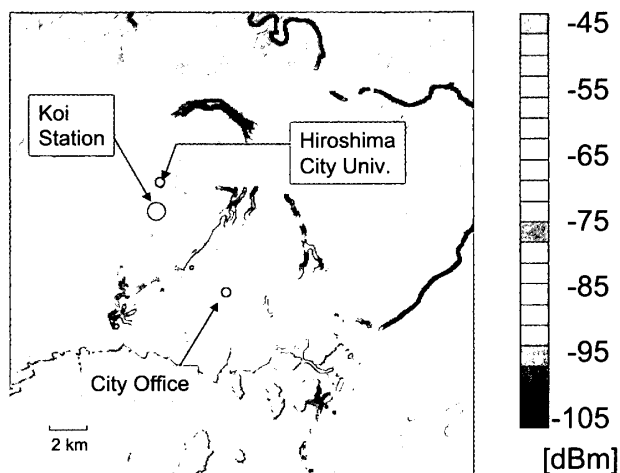
図 12 NLOS 受信レベルマップ (送信局: Koi)
