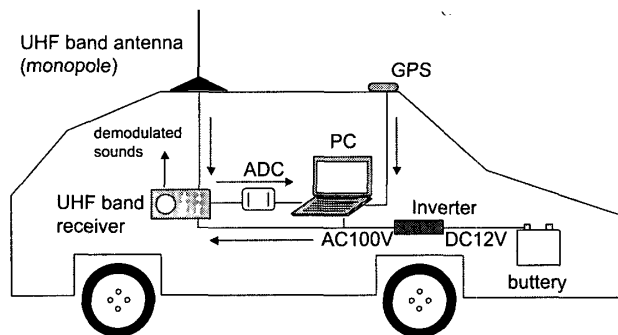
図3 移動型電波伝搬測定システム
