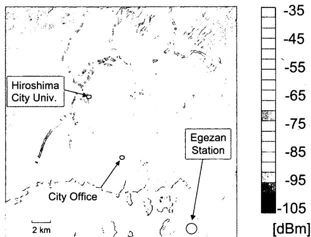
図 14 NLOS 受信レベルマップ (送信局: Egezan)
