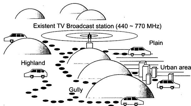
図 2 TV 放送波を用いた UHF 帯電波伝搬測定イメージ図 Fig. 2 Measurement method of UHF band radio propagation using TV broadcasting wave.
