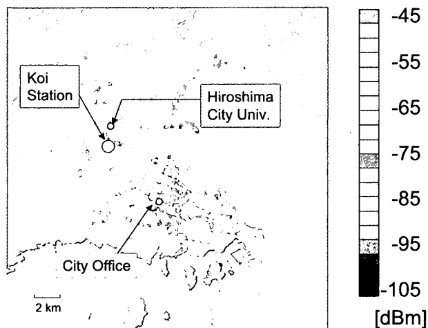
図 11 LOS 受信レベルマップ (送信局: Koi)
